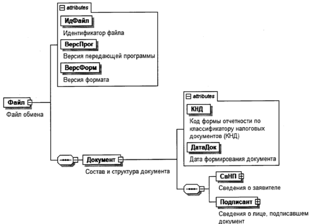
Рисунок 1. Диаграмма структуры файла обмена
