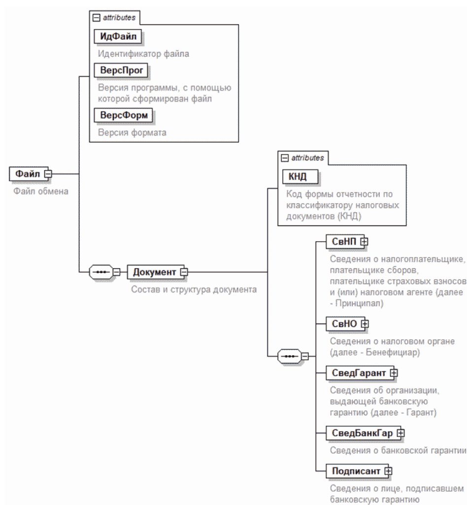
Рисунок 1. Диаграмма структуры файла обмена
