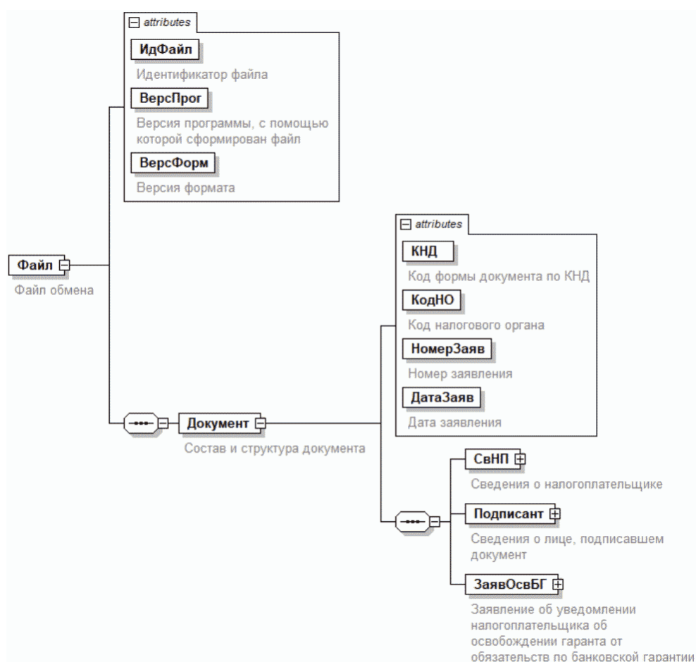
Рисунок 1. Диаграмма структуры файла обмена
