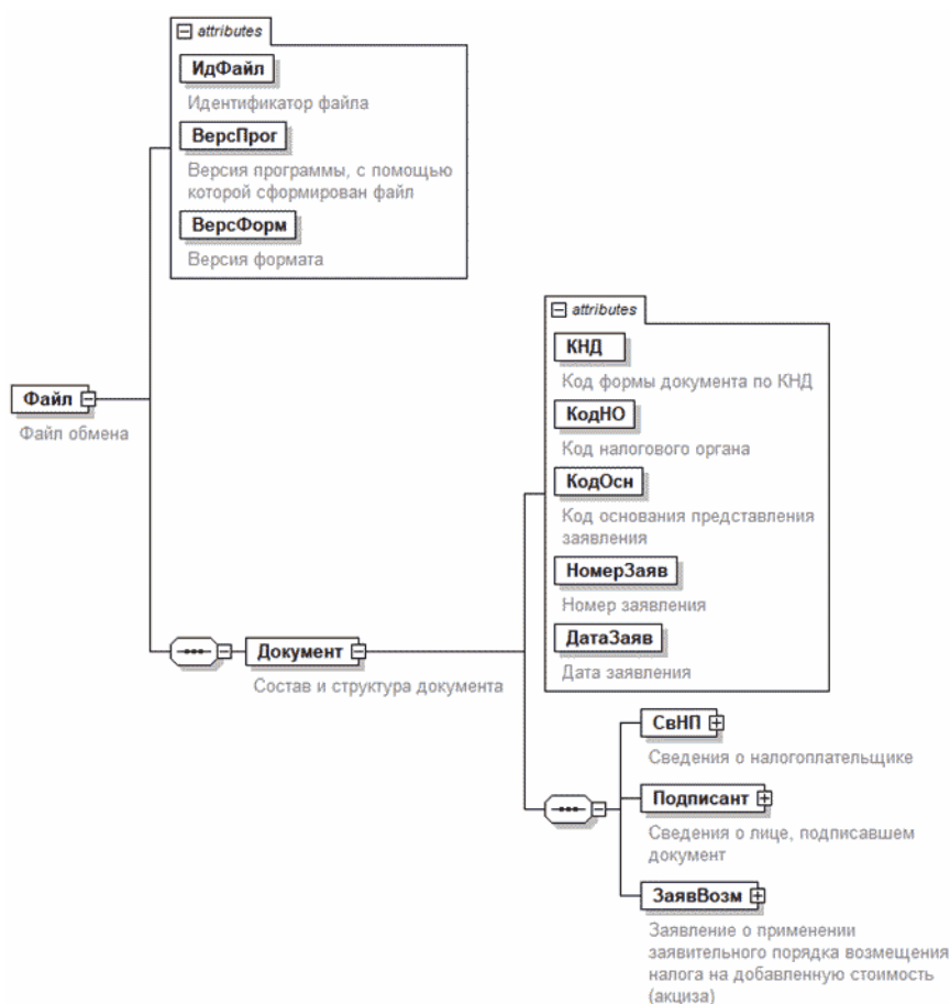
Рисунок 1. Диаграмма структуры файла обмена
